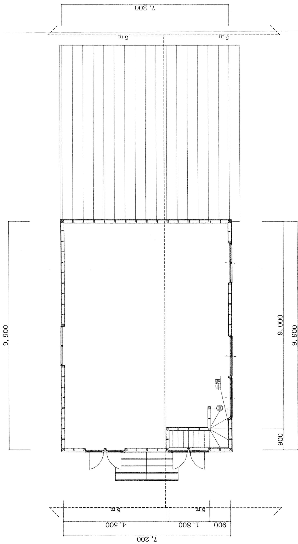
平面詳細図 2階
