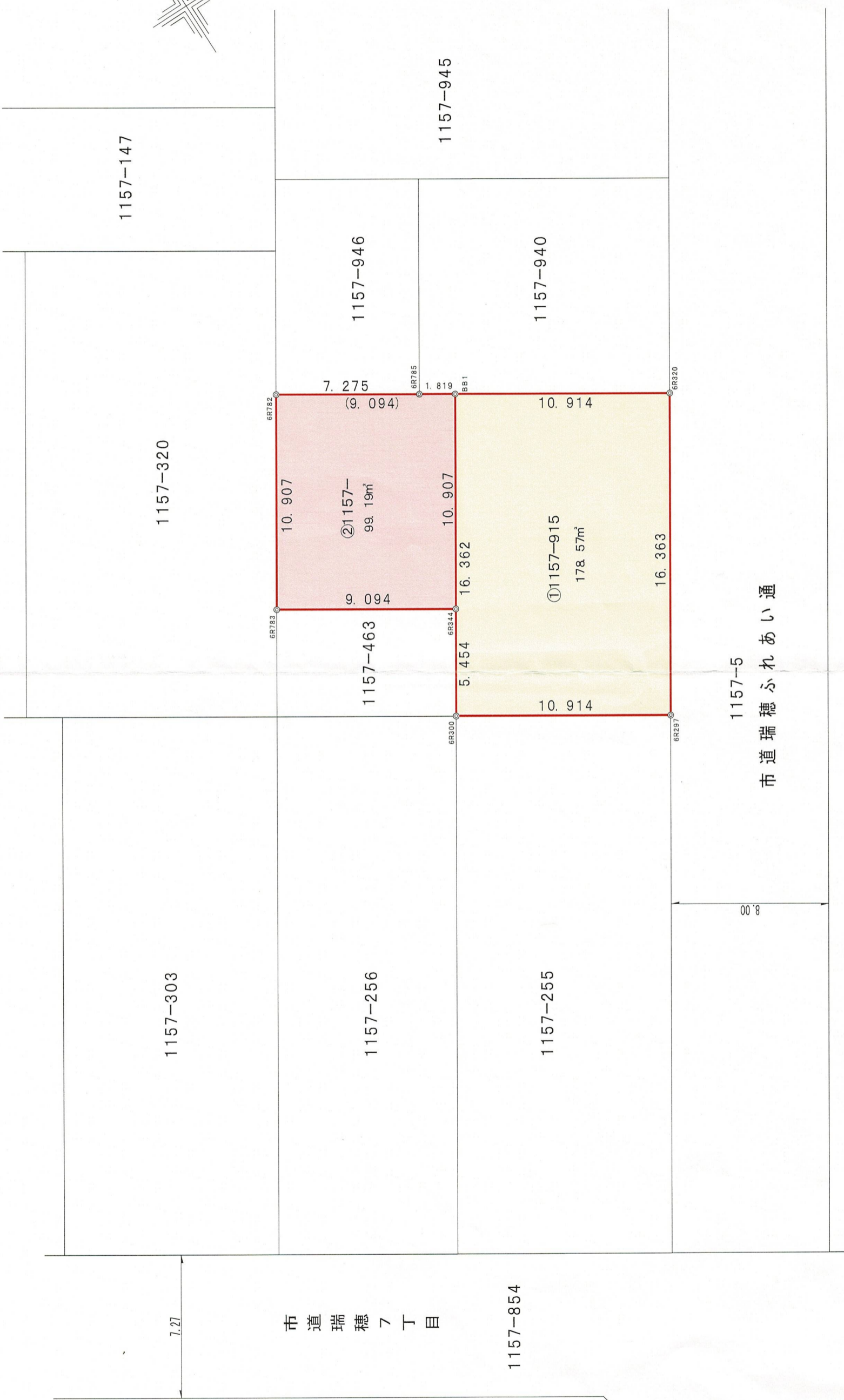
直角座標法求積表
